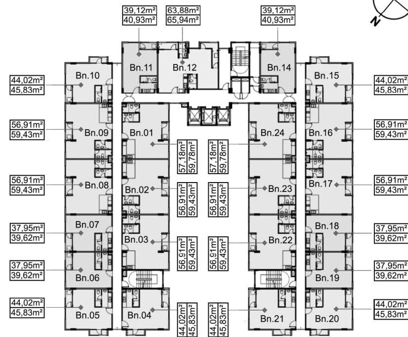
MẶT BẰNG TẦNG 3-9 (LẦU 2-8)
