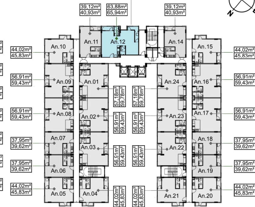
TẦNG: 3; 4; 5; 6
