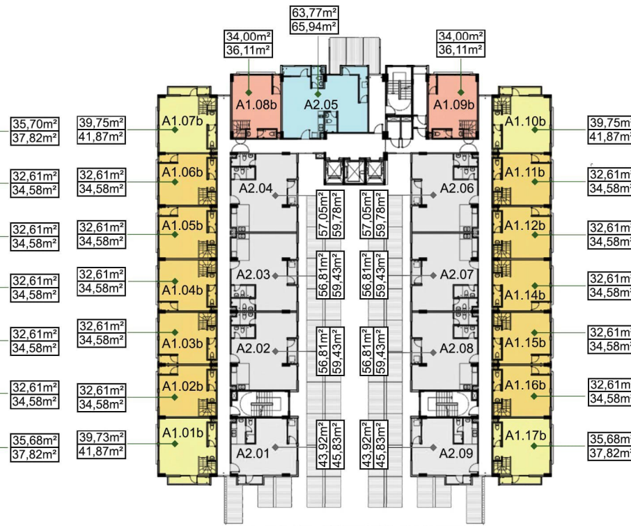
MẶT BẰNG TẦNG 2 (LẦU 1)
